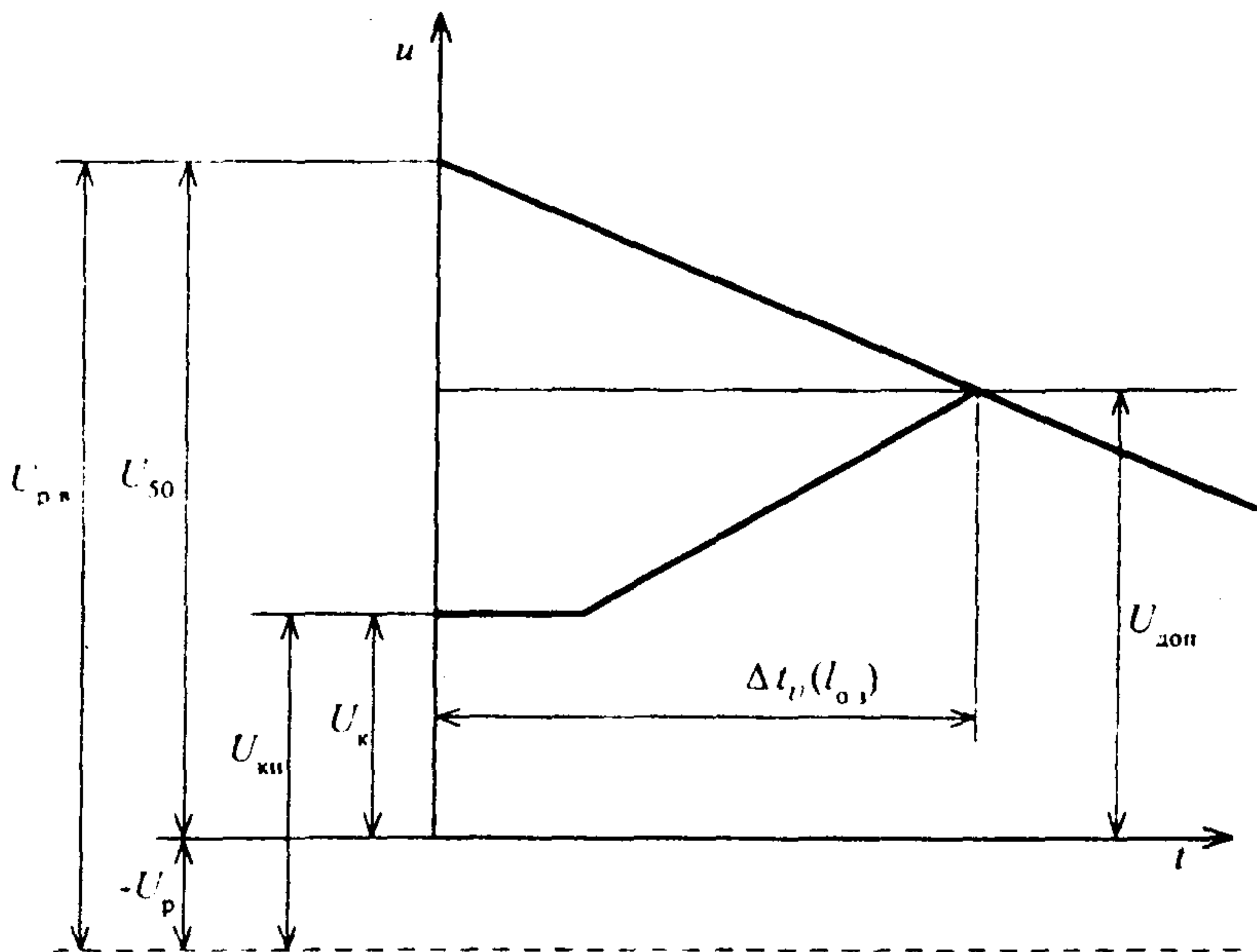
Рис. 9.4. Определение длины опасной зоны ( l_{0,3} ) по "методу бегущей волны"
