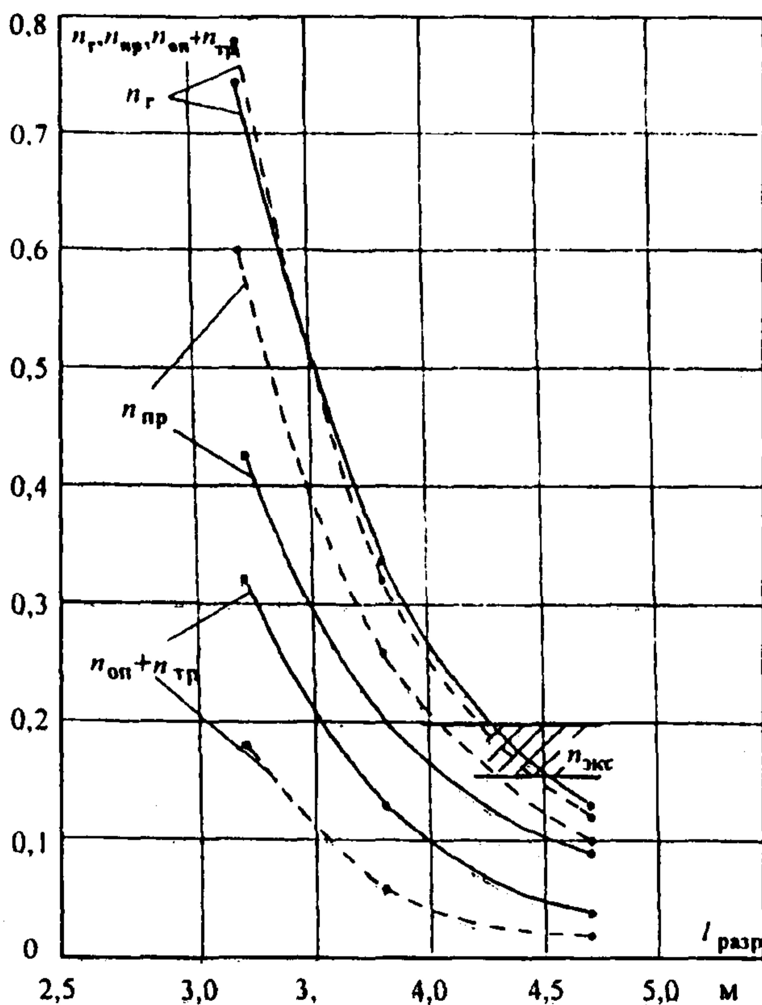
Рис. П24.1. Удельное число грозовых отключений ВЛ 500 кВ на стальных и железобетонных порталных опорах с оттяжками в зависимости от l_{\text{разр}} (на 100 км и 100 грозовых часов).
