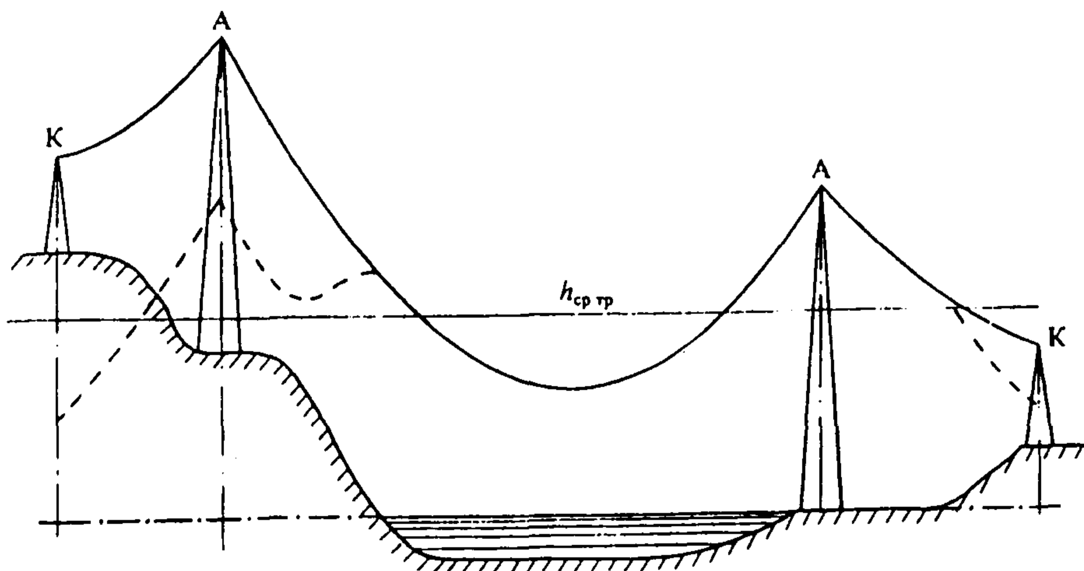
Рис. П20.1. Спрямление профиля перехода относительно уровня поверхности воды для расчета его грозопоражаемости: — действительное расположение троса; - - - - - расчетное расположение троса (после спрямления профиля перехода)
