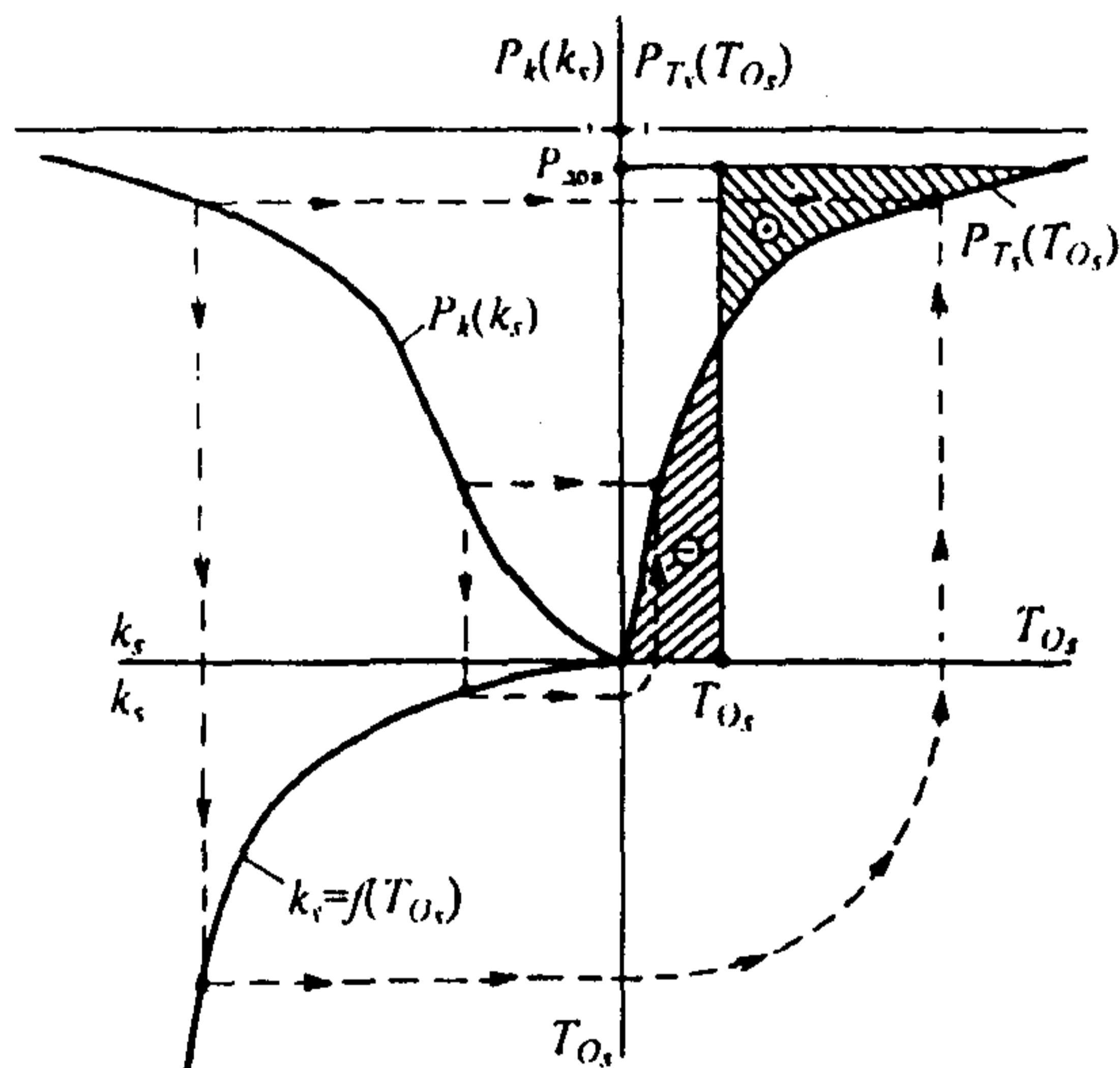
Рис. Пб.6. Графическое построение статистического распределения P_{TS}(T_{OS}) и математического ожидания \bar{T}_{OS} ресурса, расходуемого в одной коммутации S -го типа, при заданной доверительной вероятности P_{дов}
