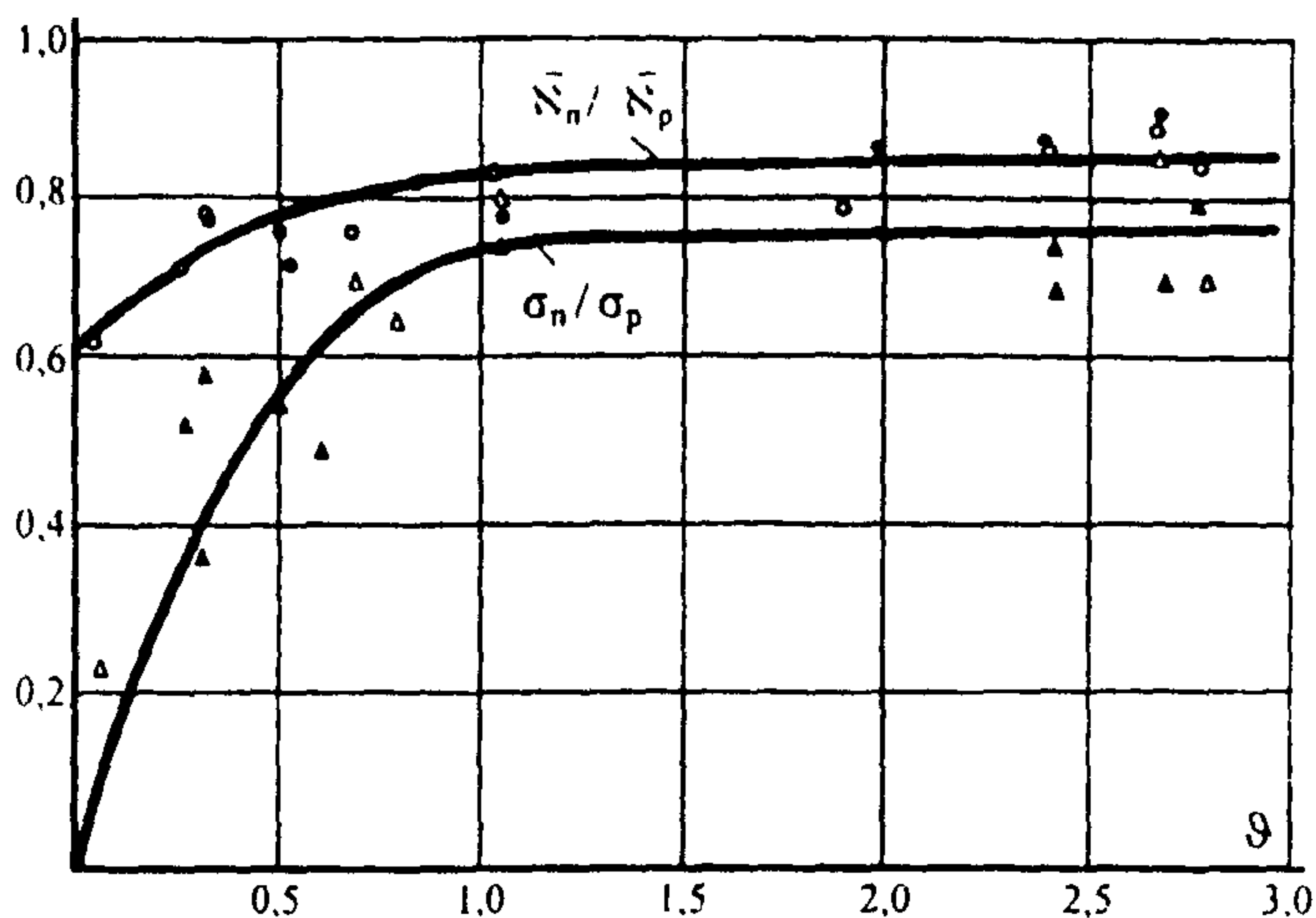
Рис. Пб.1. Зависимость отношений \bar{N}_n / \bar{N}_p и \sigma_n / \sigma_p от параметра Q : кружки, треугольники – опытные точки, соответственно \bar{N}_n / \bar{N}_p и \sigma_n / \sigma_p ; белые и черные значки, соответственно ВЛ без заряда и предварительно заряженные
