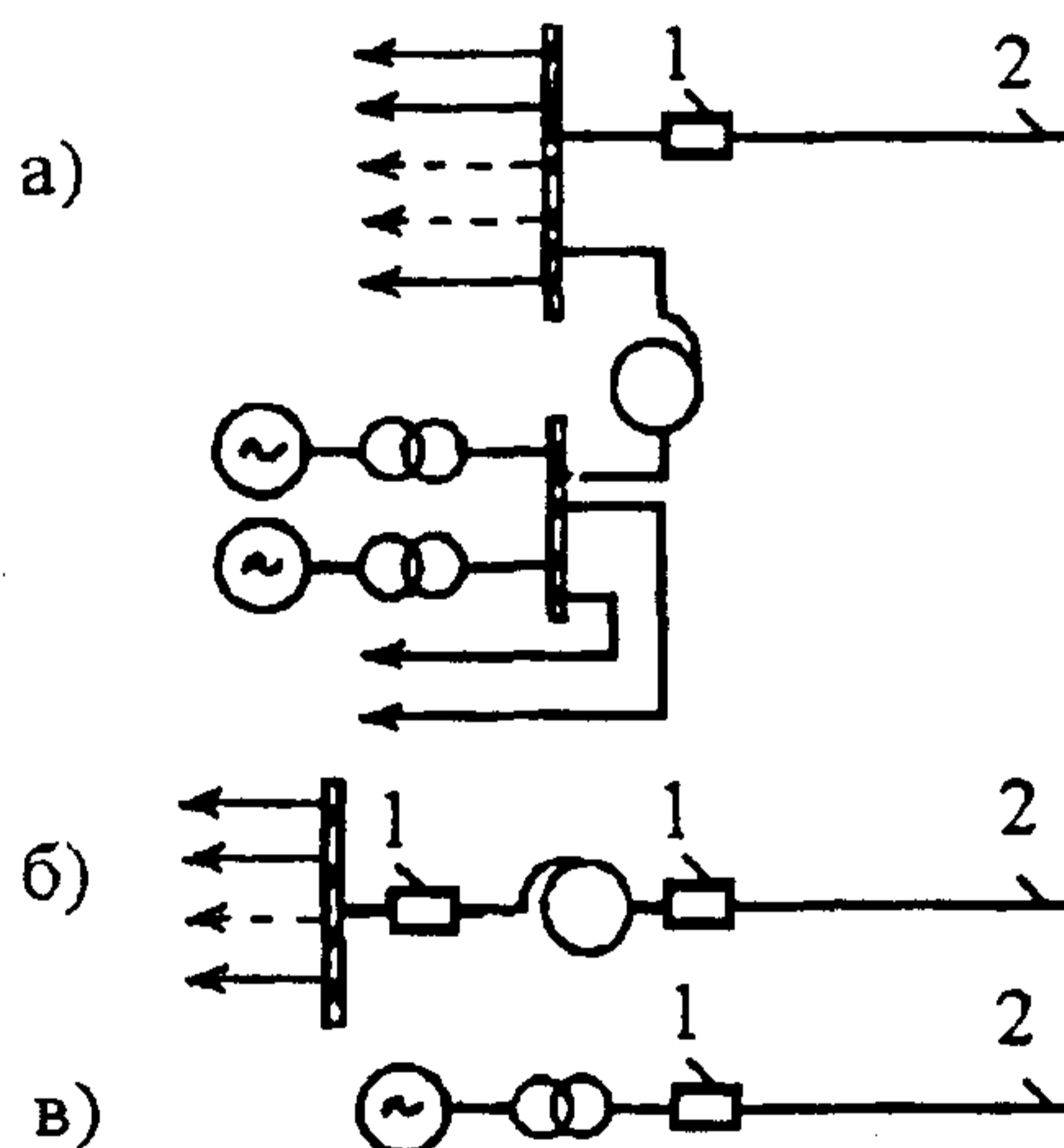
Рис. П.2.6. Принципиальные схемы источника питания.
