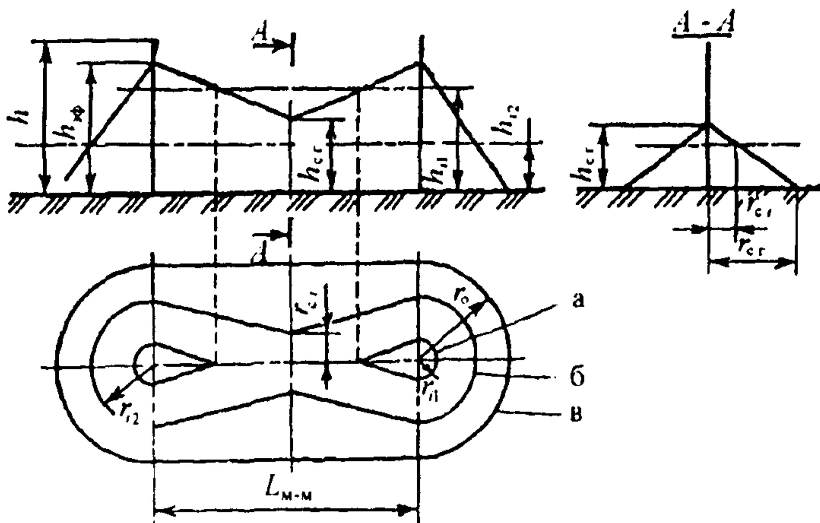
Рис. П29.2. Зоны защиты двух стержневых молниеотводов одинаковой высоты: а – граница зоны защиты на уровне h_{и1} ; б – то же на уровне h_{и2} ; в – то же, на уровне земли (при L_{м-м} \leq 2h )
