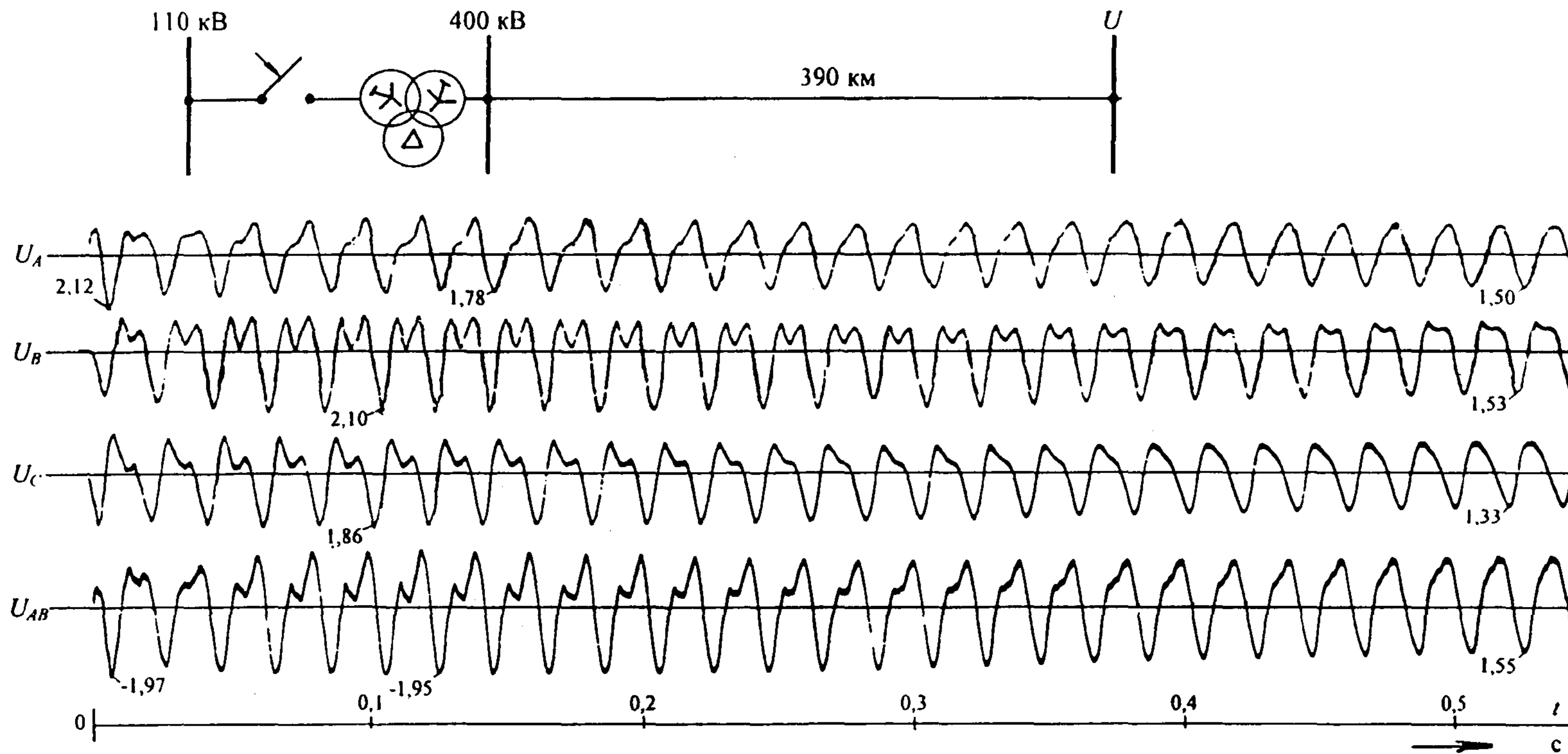
Рис. 2.3.а. Перенапряжения на частоте 100Гц при переходном феррорезонансе. ВЛ Ногинск-Арзамас
