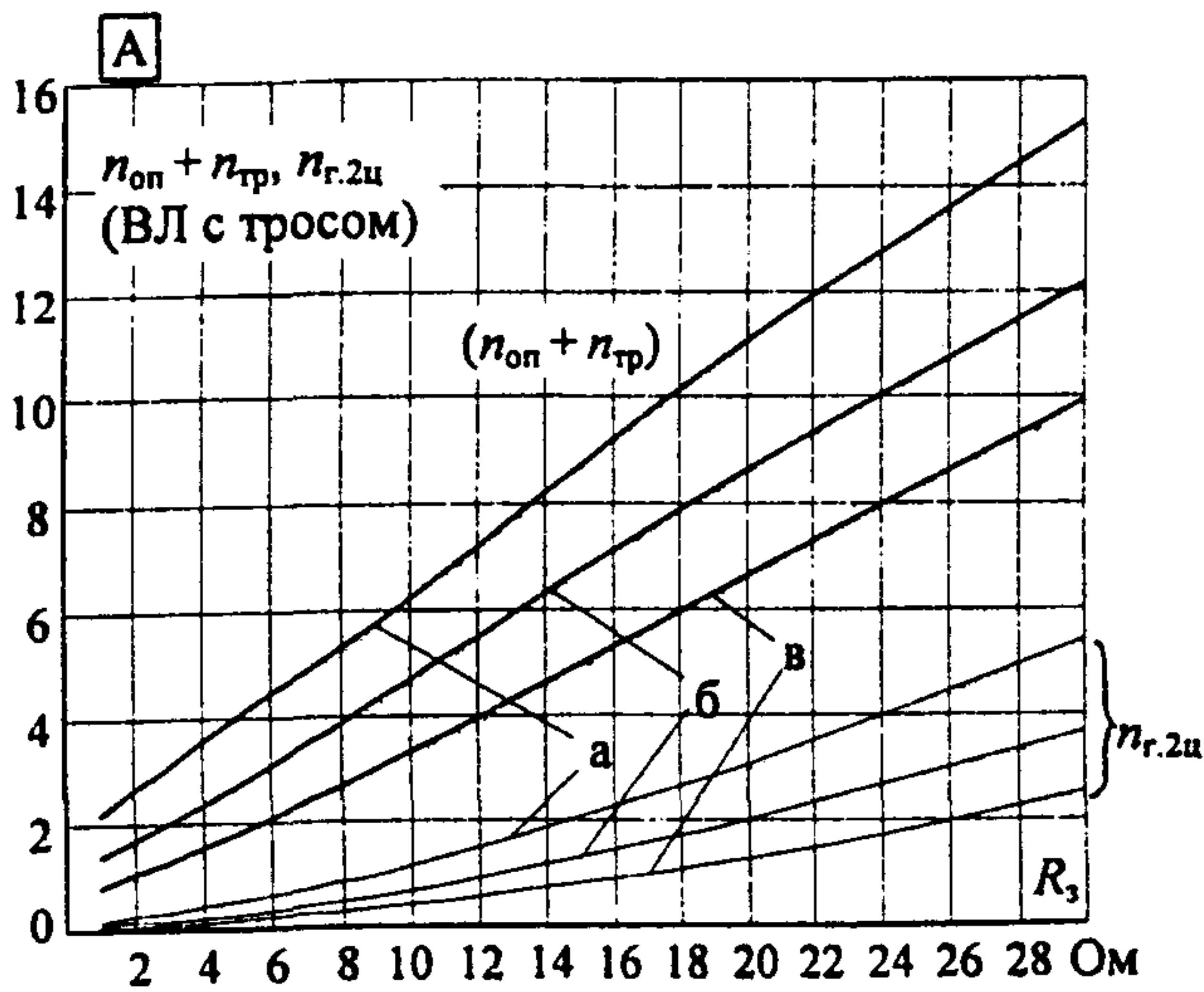
Рис. П23.4. Удельное число грозовых отключений ВЛ 110 кВ на двухцепных железобетонных опорах с одним тросом при различной линейной изоляции: а) 8 ПС70Е l_{разр}=1,02 м; б) 9 ПС70Е l_{разр}=1,14 м; в) 10 ПС70Е l_{разр}=1,27 м (на 100 км и 100 грозовых часов); — ВЛ с тросом; - - - - ВЛ без троса
