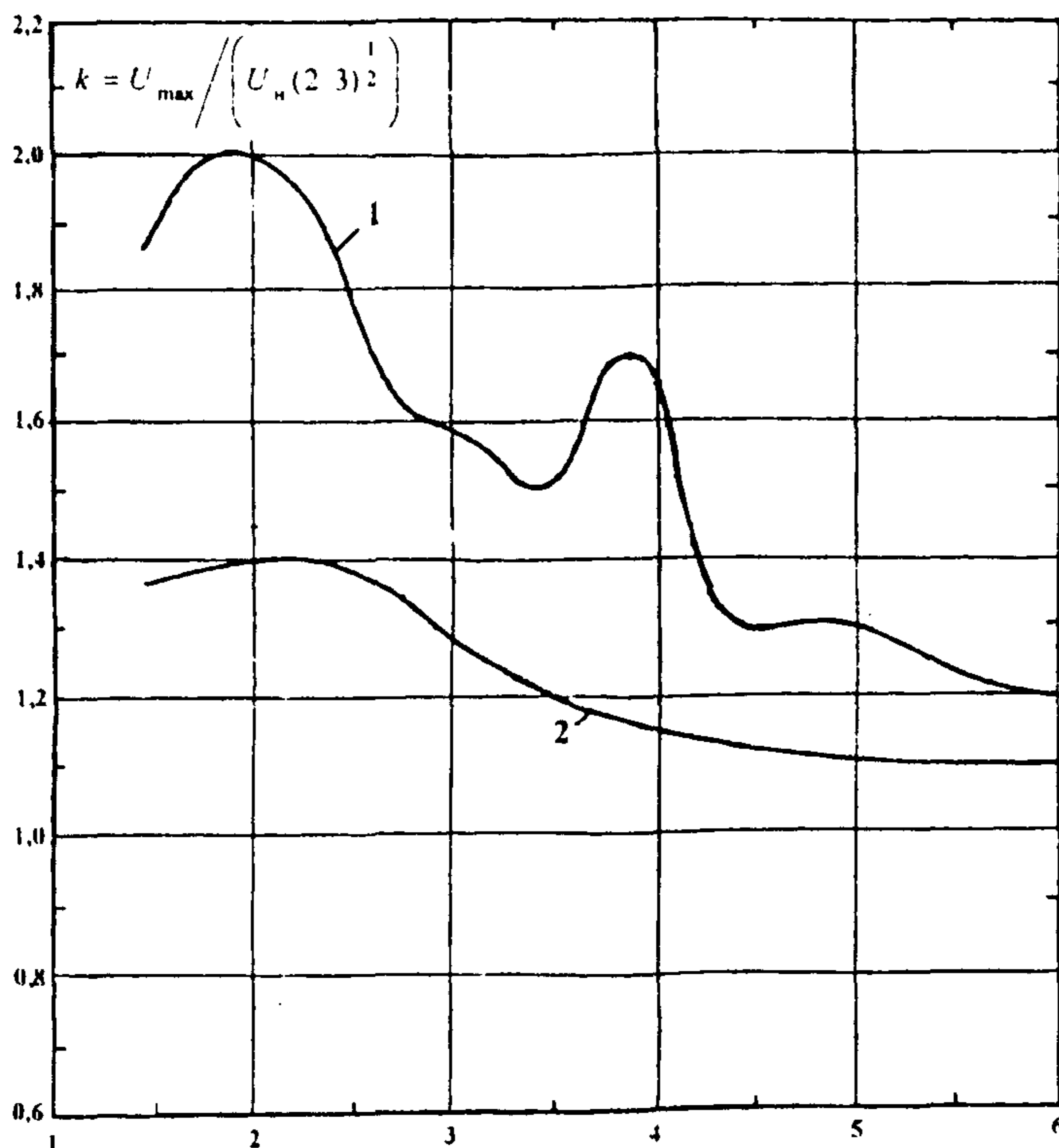
Рис. П2.7. Перенапряжения при переходном феррорезонансе.
