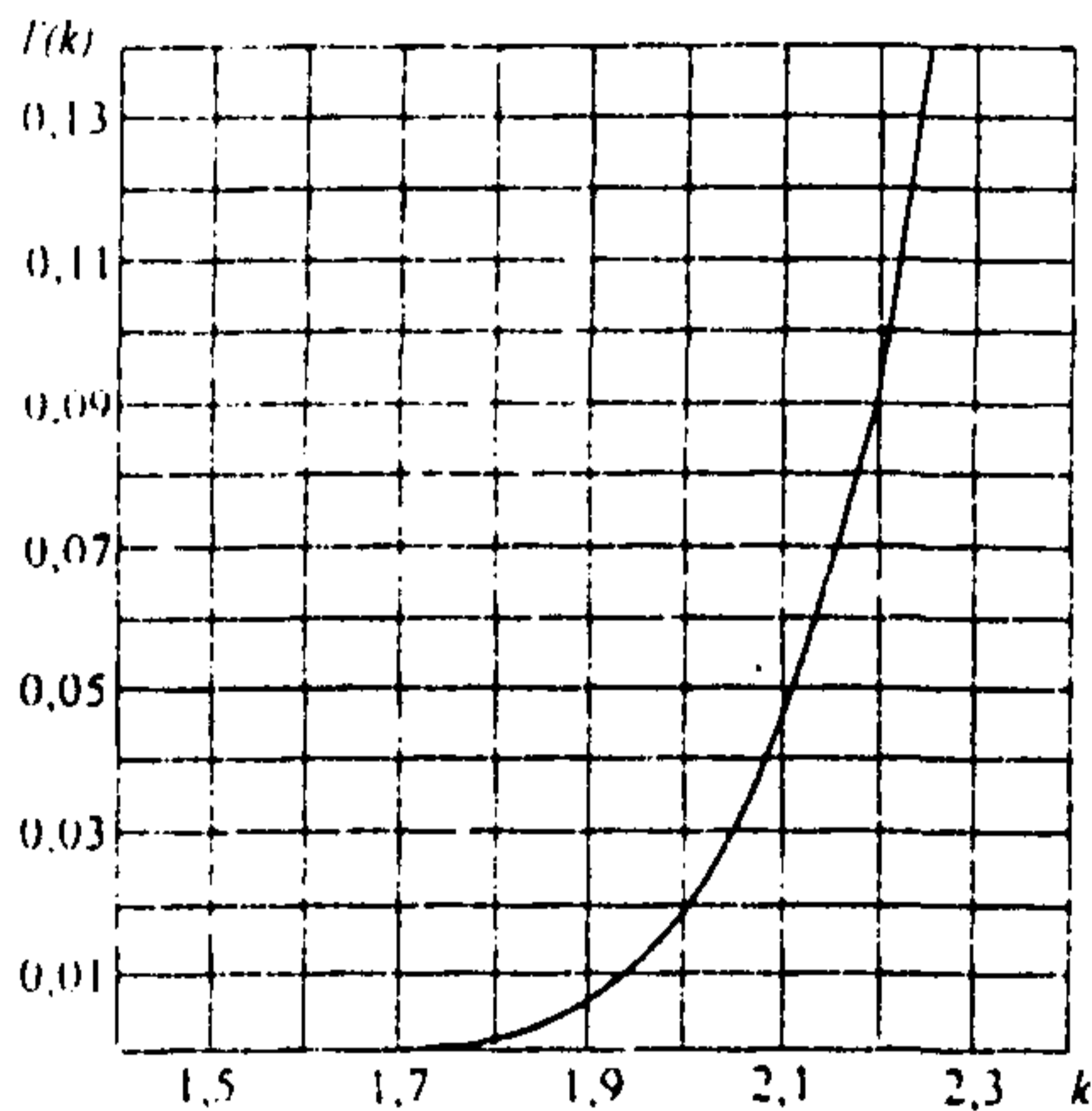
Рис. П8.2. Зависимость T(k) для ОПН-750 кВ
