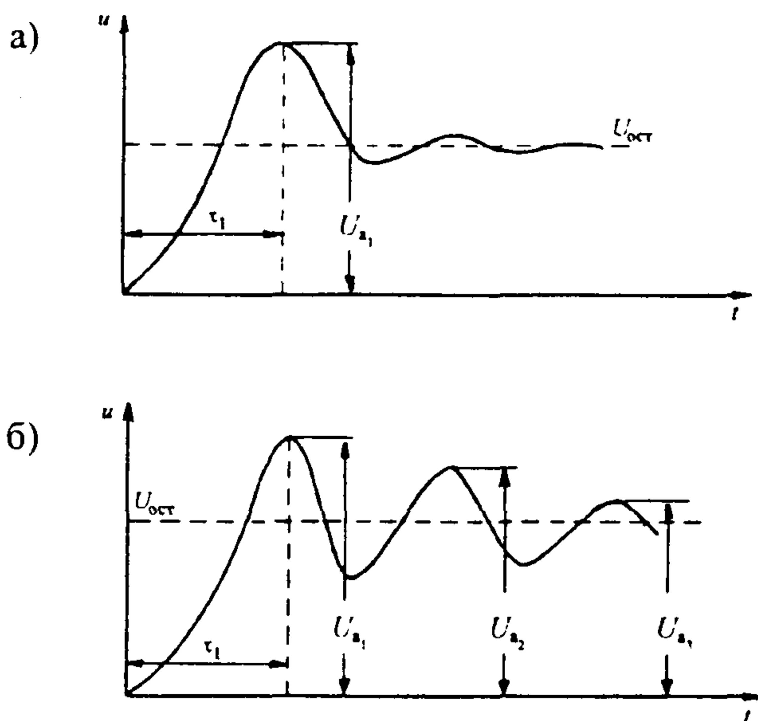
Рис. 9.1. Характерная форма грозовых перенапряжений на подстанционном оборудовании:
