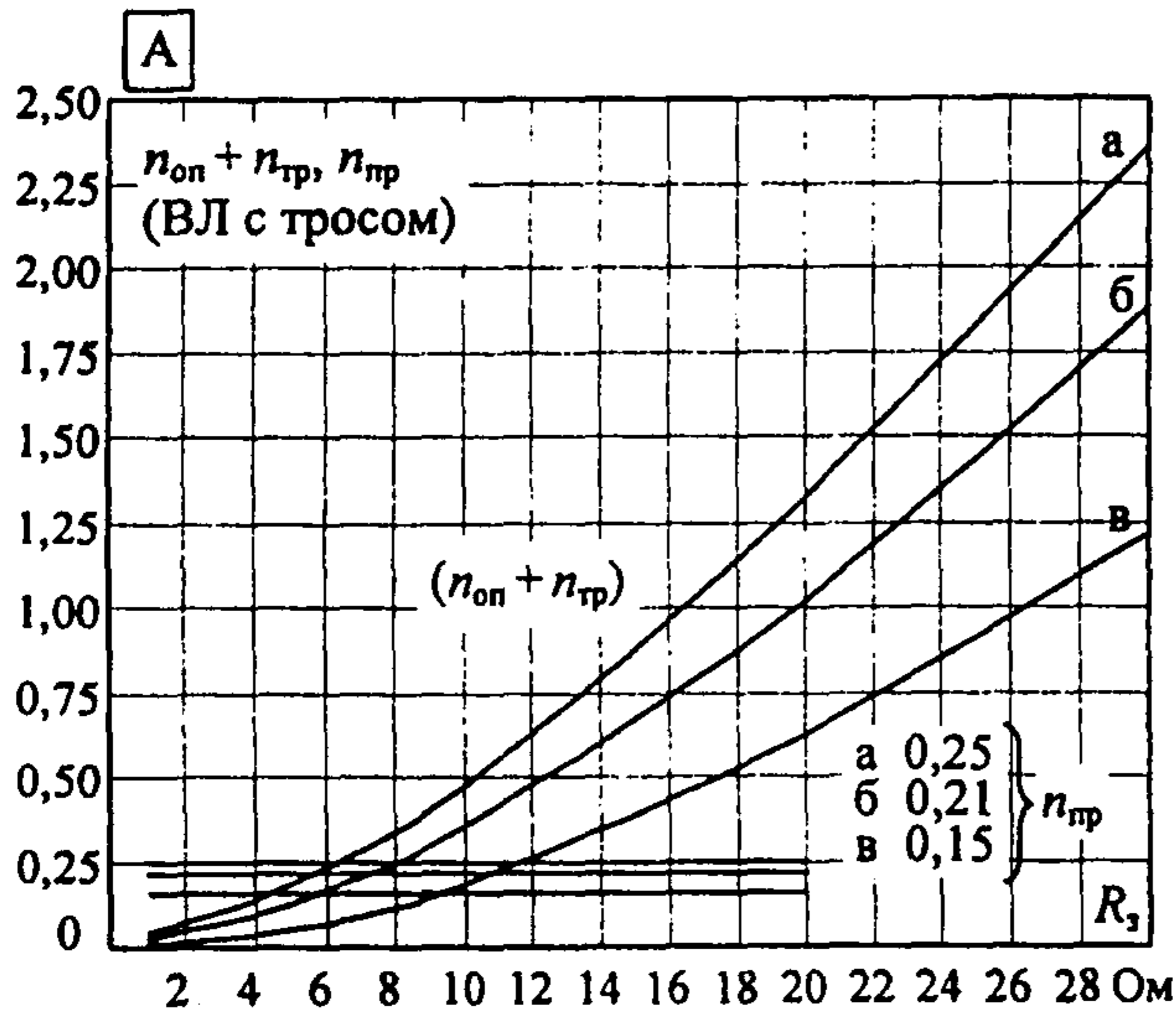
Рис. П23.16. Удельное число грозových отключений ВЛ 220 кВ на одноцепных порталных опорах с двумя тросами при различной линейной изоляции: а) 14 ПС70Е l_{разр}=1,78 м; б) 15 ПС70Е l_{разр}=1,91 м; в) 17 ПС70Е l_{разр}=2,16 м (на 100 км и 100 грозových часов); — ВЛ с тросом; - - - - ВЛ без троса
