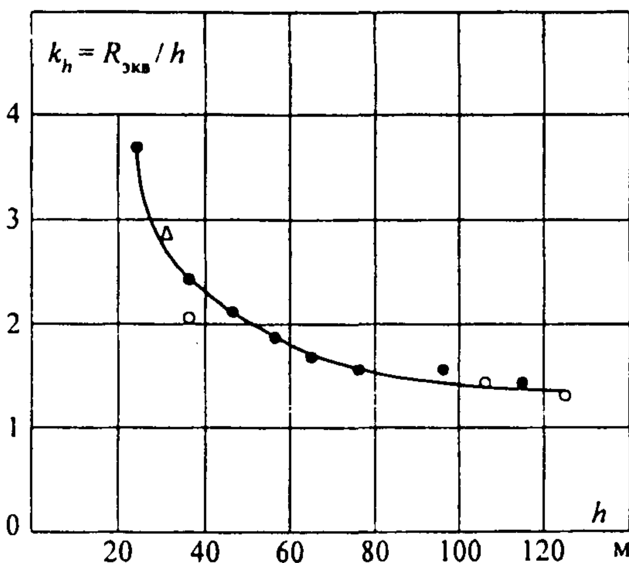
Рис. 6.10. Зависимость отношения ширины полосы, с которой ВЛ собирает боковые разряды молний с одной стороны от ВЛ ( R_{экв} ), к высоте опор по данным польских исследований: ● бывшая Чехословакия; ○ Польша; Δ Украина
