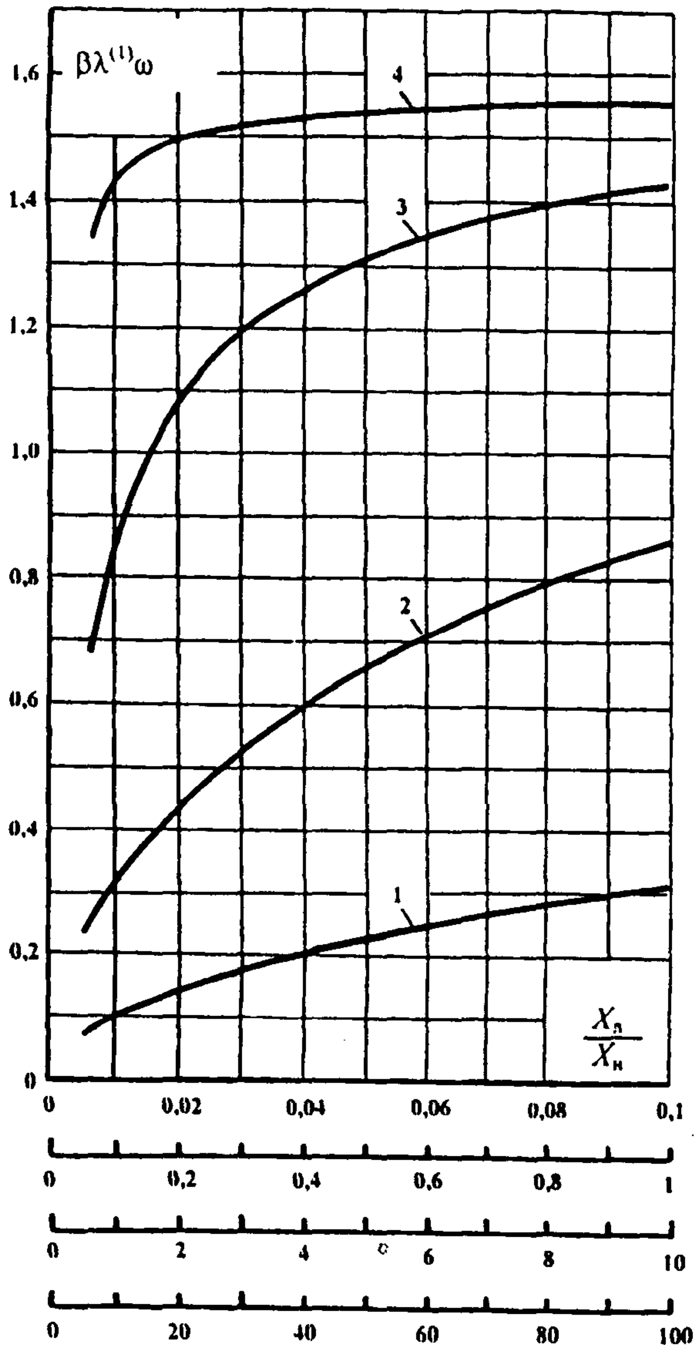
Рис. ПЗ.1. 1 – для X_n / X_1 = 0,01-0,1 ; 2 – для X_n / X_1 = 0,1-1,0 ; 3 – для X_n / X_1 = 1,0-10 ; 4 – для X_n / X_1 = 10-100 . \beta_{(1)} – наименьшая собственная частота в долях промышленной частоты; \lambda^{(1)} – волновая длина линии в радианах (см. табл. П2.1.; табл.П2.2. и рис. П2.1. Приложения 2); l – длина линии, км; X_1 – сопротивление предвключенной индуктивности на промышленной частоте, Ом; X_n – индуктивное сопротивление линии, Ом, равное 314 \cdot l \cdot L_n ; ( L_n – Гн/км.)
