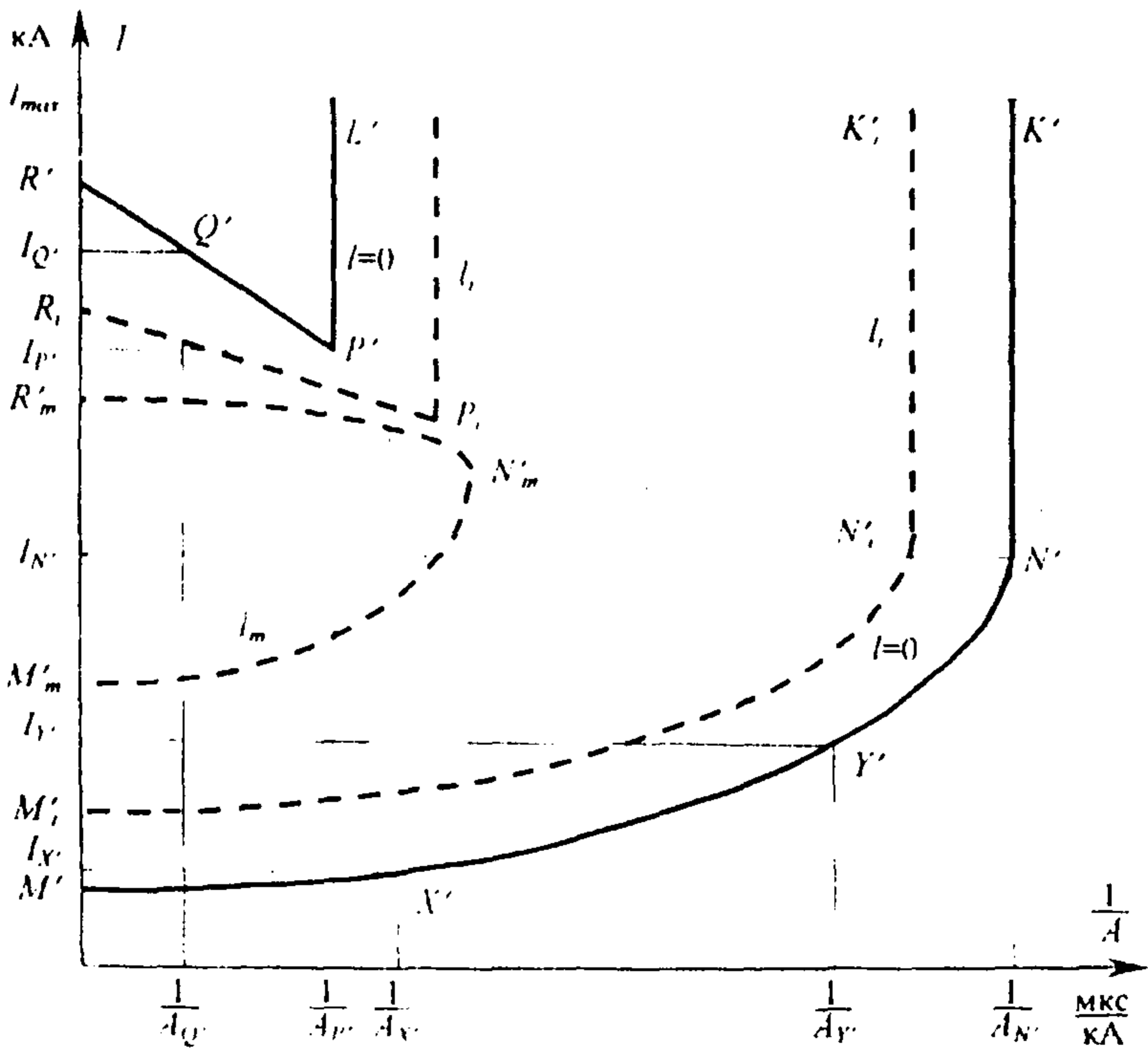
Рис. П.33.3. Область существования параметров опасных волн в координатах I , 1/A
