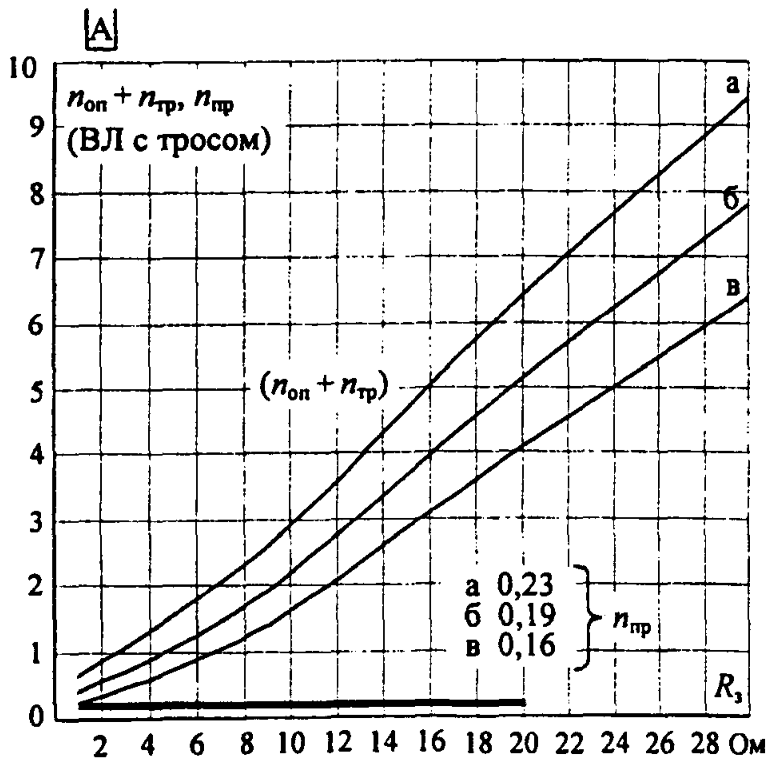
Рис. П23.7. Удельное число грозových отключений ВЛ 150 кВ на одноцепных железобетонных опорах с одним тросом при различной линейной изоляции: а) 10 ПС70Е l_{разр} = 1,27 м; б) 11 ПС70Е l_{разр} = 1,40 м; в) 13 ПС70Е l_{разр} = 1,65 м (на 100 км и 100 грозových часов); — ВЛ с тросом; - - - - ВЛ без троса
