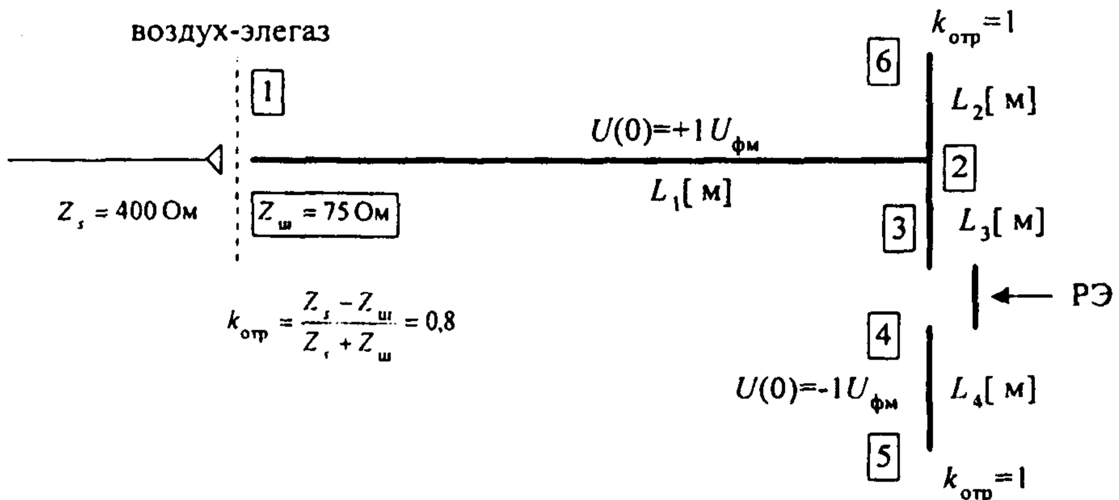
Рис. 3.2. Фрагмент компоновки полуволновой схемы КРУЭ. РЭ – коммутирующий элегазовый разъединитель
