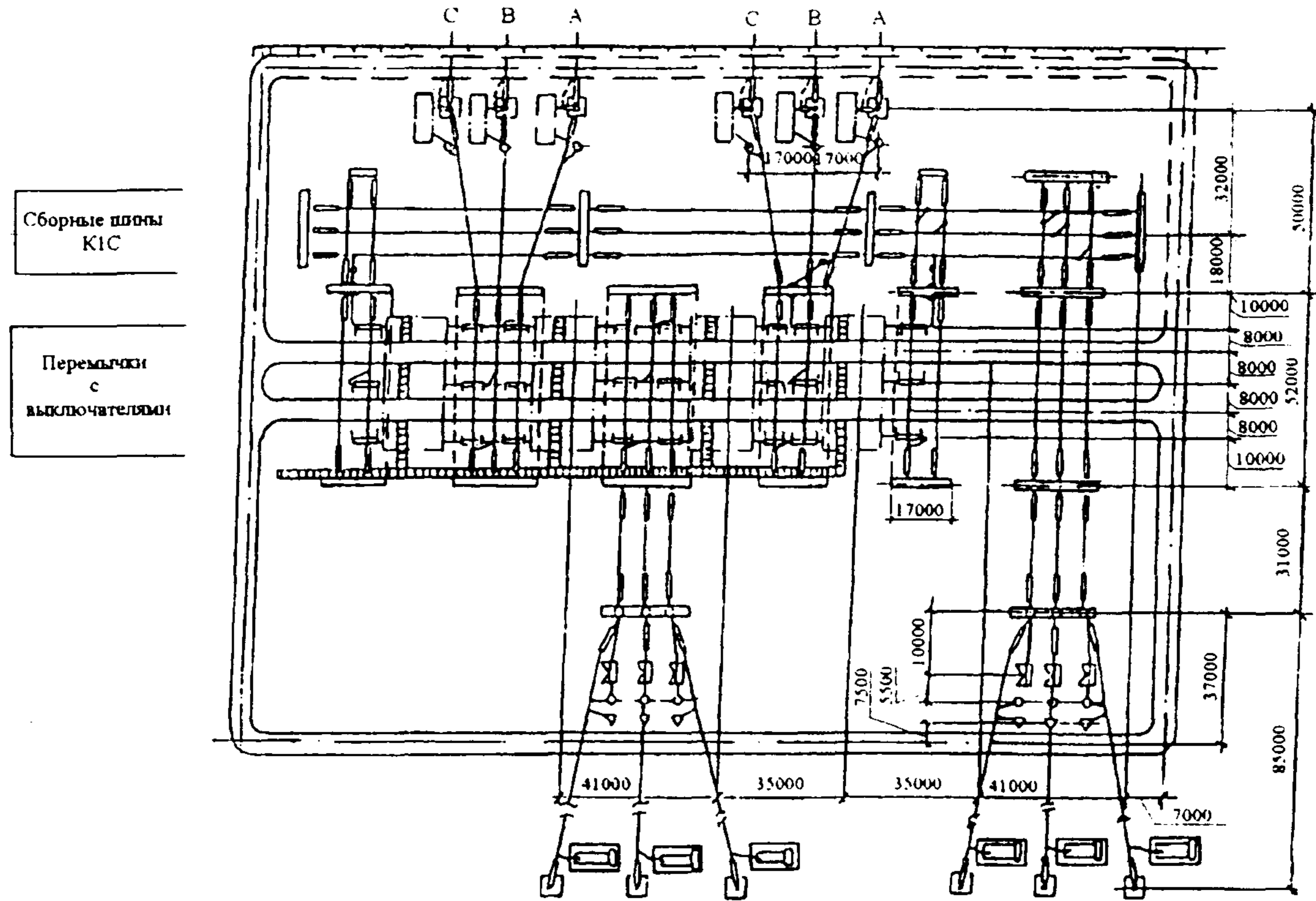
Рис. П30.2. План ПС
