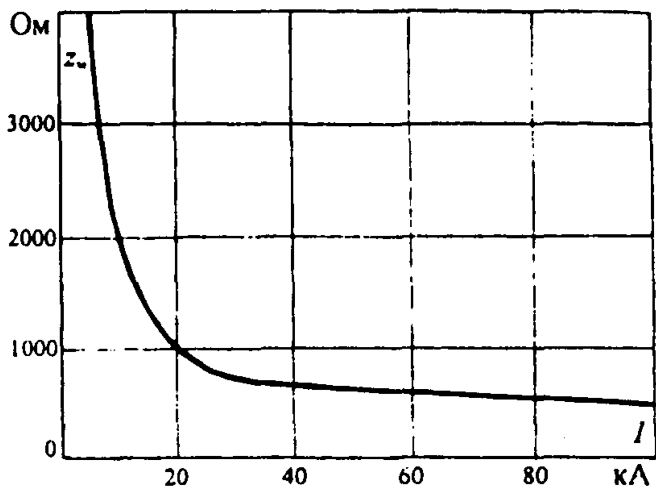
Рис. 6.7. Зависимость эквивалентного сопротивления канала от тока молнии
