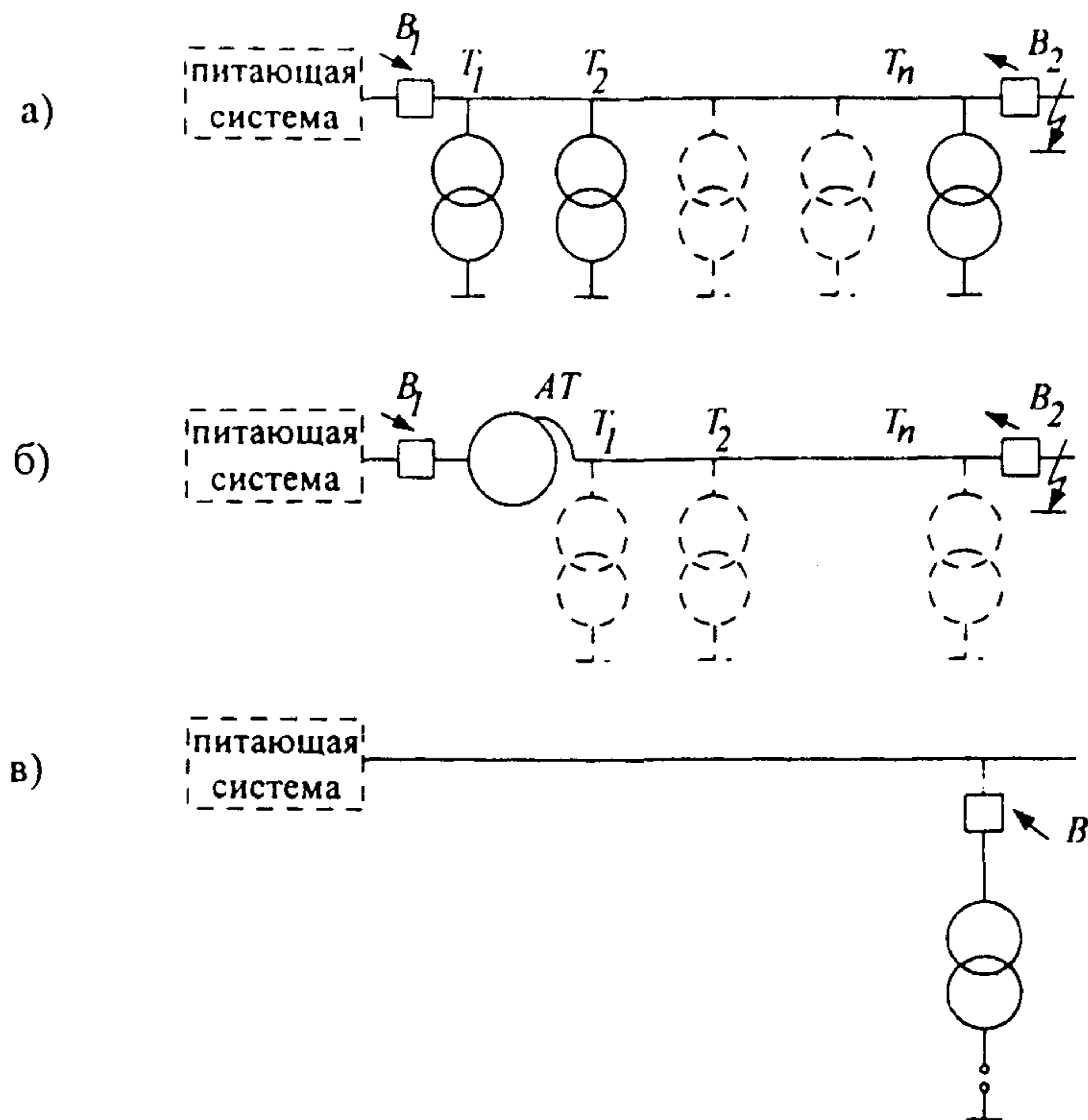
Рис. 1. 1. Схемы электропередач, подверженных переходному феррорезонансу
