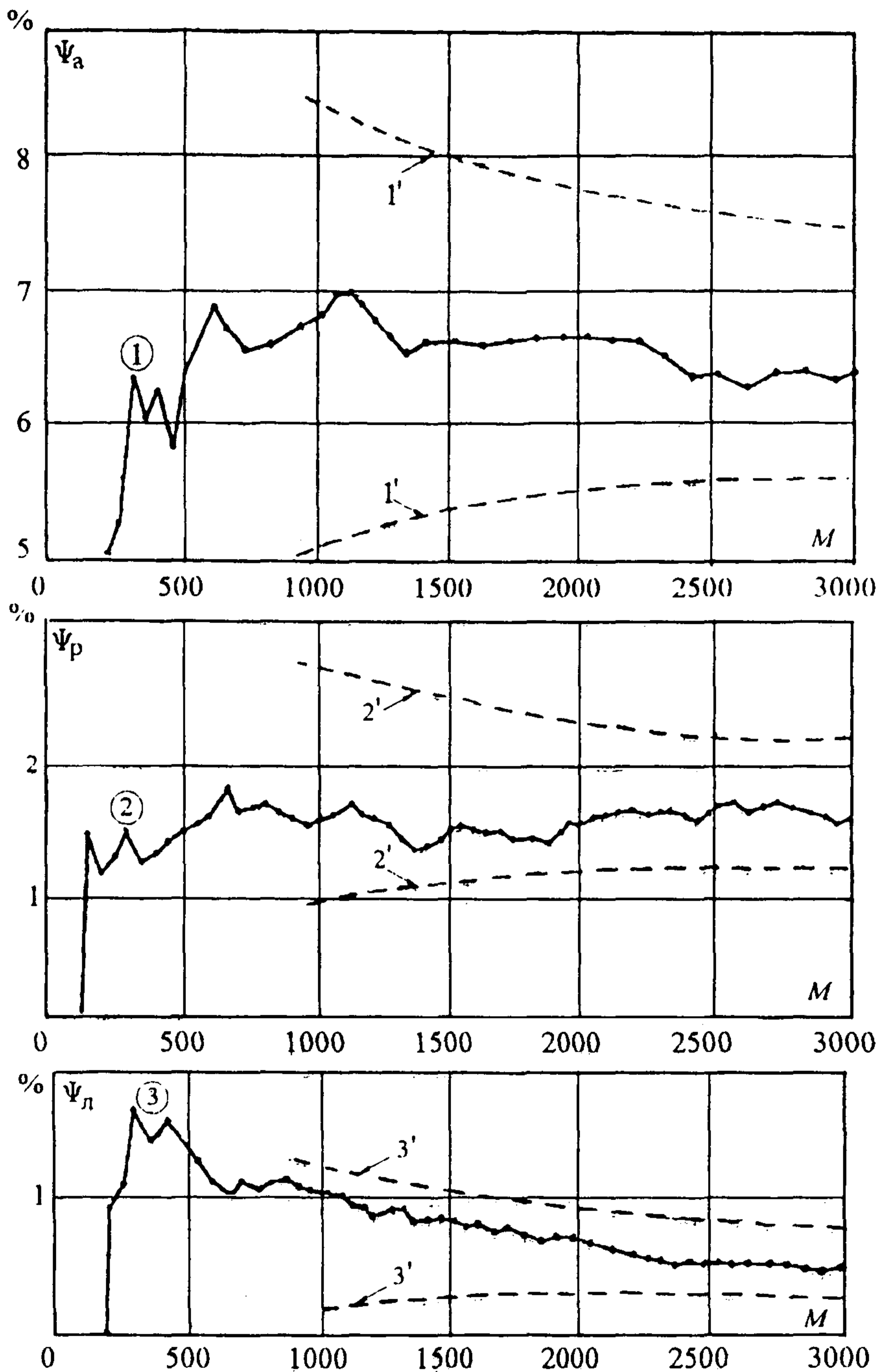
Рис. П32.1. Доля опасных волн (—•—•—•—) и ее доверительные интервалы (---) в зависимости от числа статистических испытаний для трех точек ПС: 1 – автотрансформатор ( \psi_a и 1'-1'); 2 – реактор ( \psi_p и 2'-2'); 3 – линейный выключатель ( \psi_n и 3'-3')
