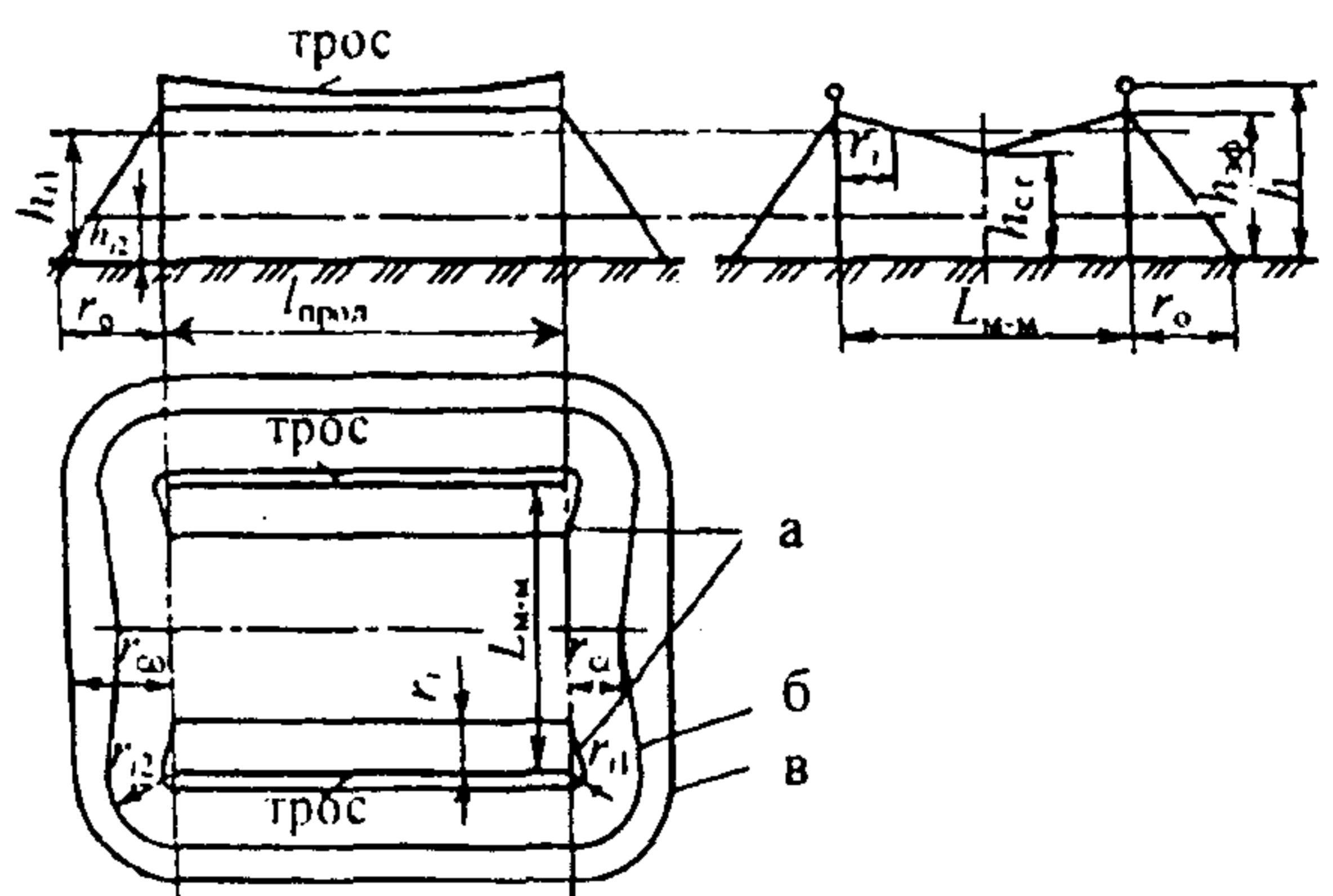
Рис. П29.6. Зоны защиты системы двух тросовых молниеотводов одинаковой высоты: а – граница зоны защиты на уровне h_1 ; б – то же, на уровне h_2 ; в – то же, на уровне земли
