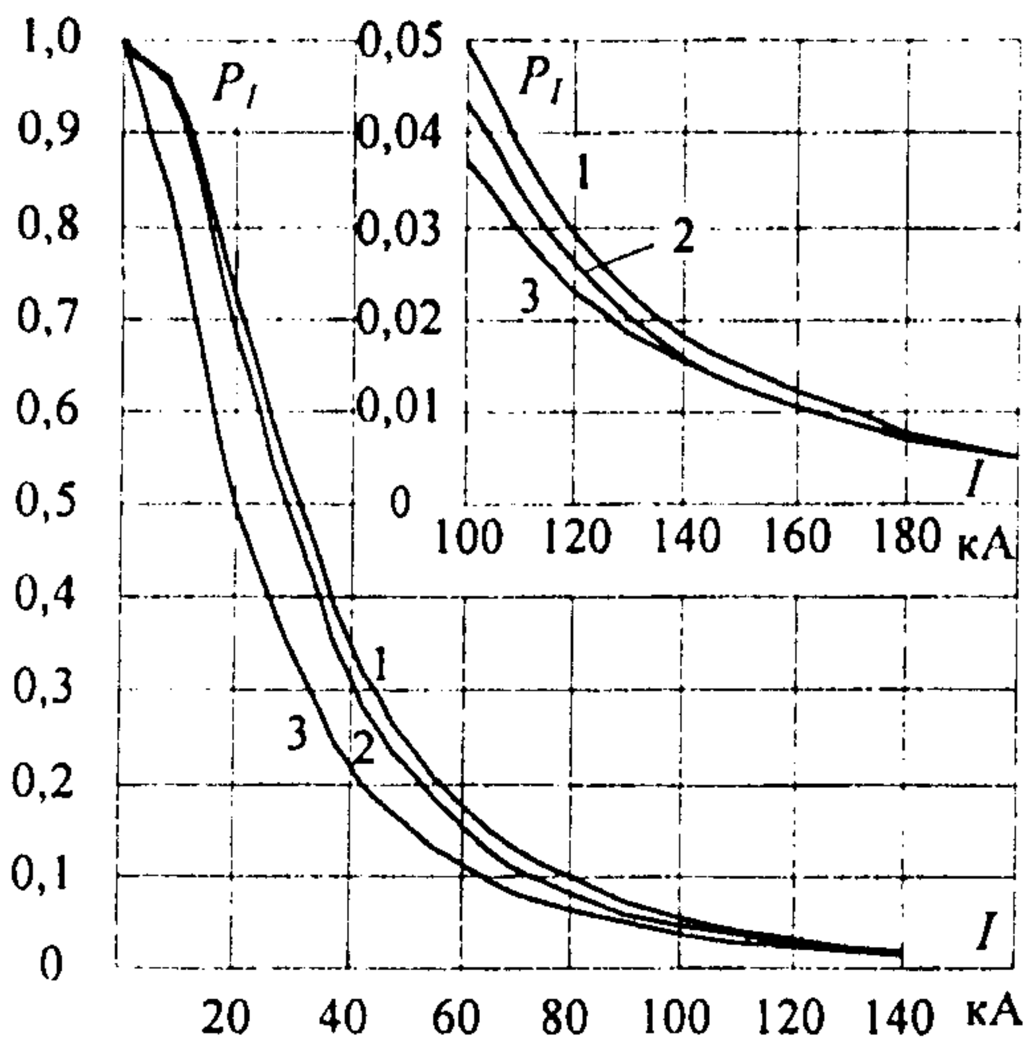
Рис. 6.5. Распределение амплитуды тока первых импульсов многократного разряда молнии: 1 – обобщенное распределение по результатам измерений преимущественно на башнях (рекомендация Исследовательского комитета № 33 СИГРЭ); 2 – по измерениям на ВЛ ( h_{\text{оп}} до 45 м); 3 – по измерениям на ВЛ ( h_{\text{оп}} до 20 м)
