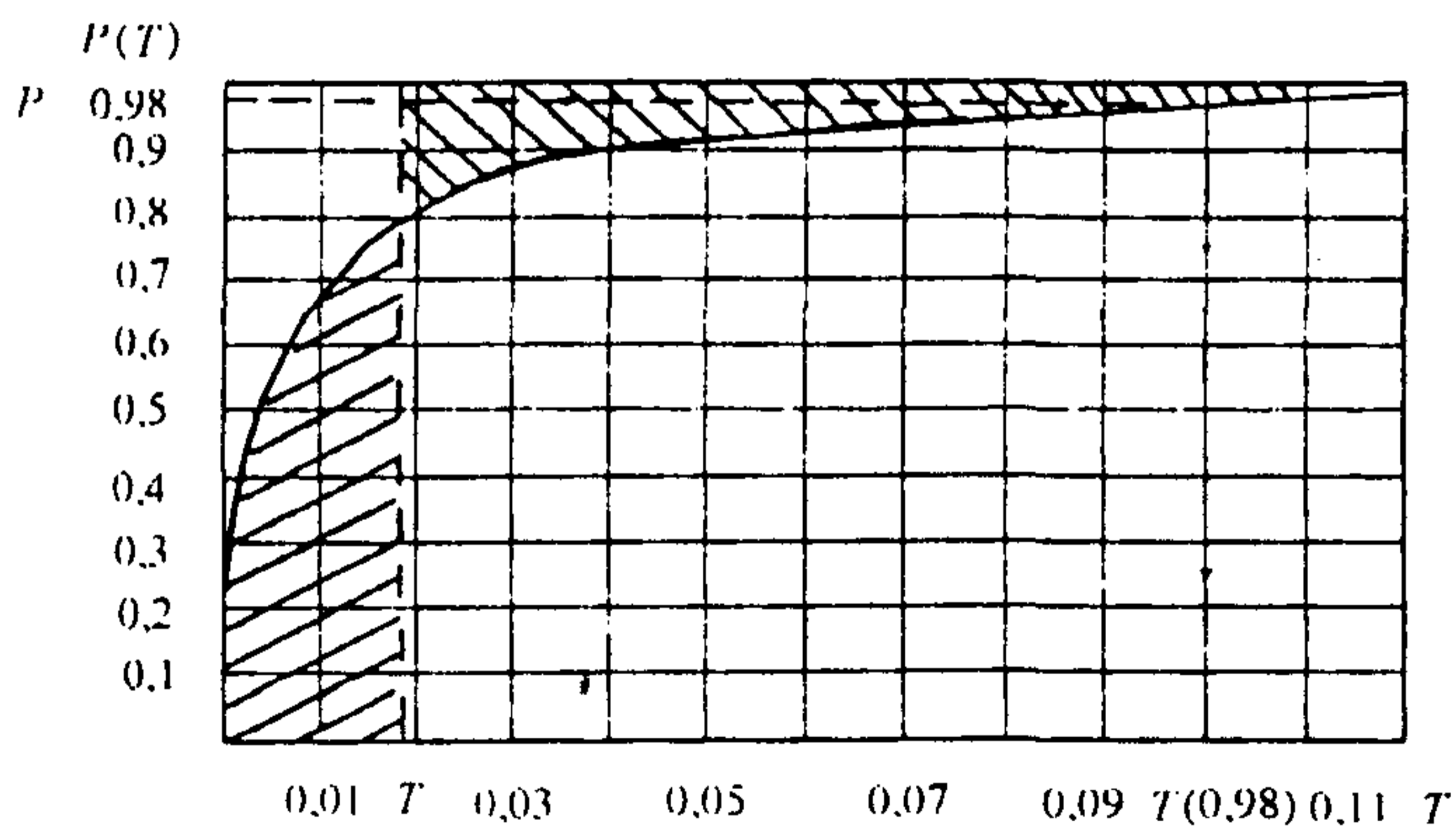
Рис. П8.3. Зависимость P(T) для коммутации планового включения. Зависимость строится на основании кривых рис. П8.1 и П8.2. Например: вероятности P = 0,8 на рис. П8.1 соответствует k = 2 , этому значению k на кривой рис. П8.2 соответствует T = 0,002 . Следовательно, на рис. П8.3 искомая точка будет иметь координаты P = 0,8 , T = 0,02
