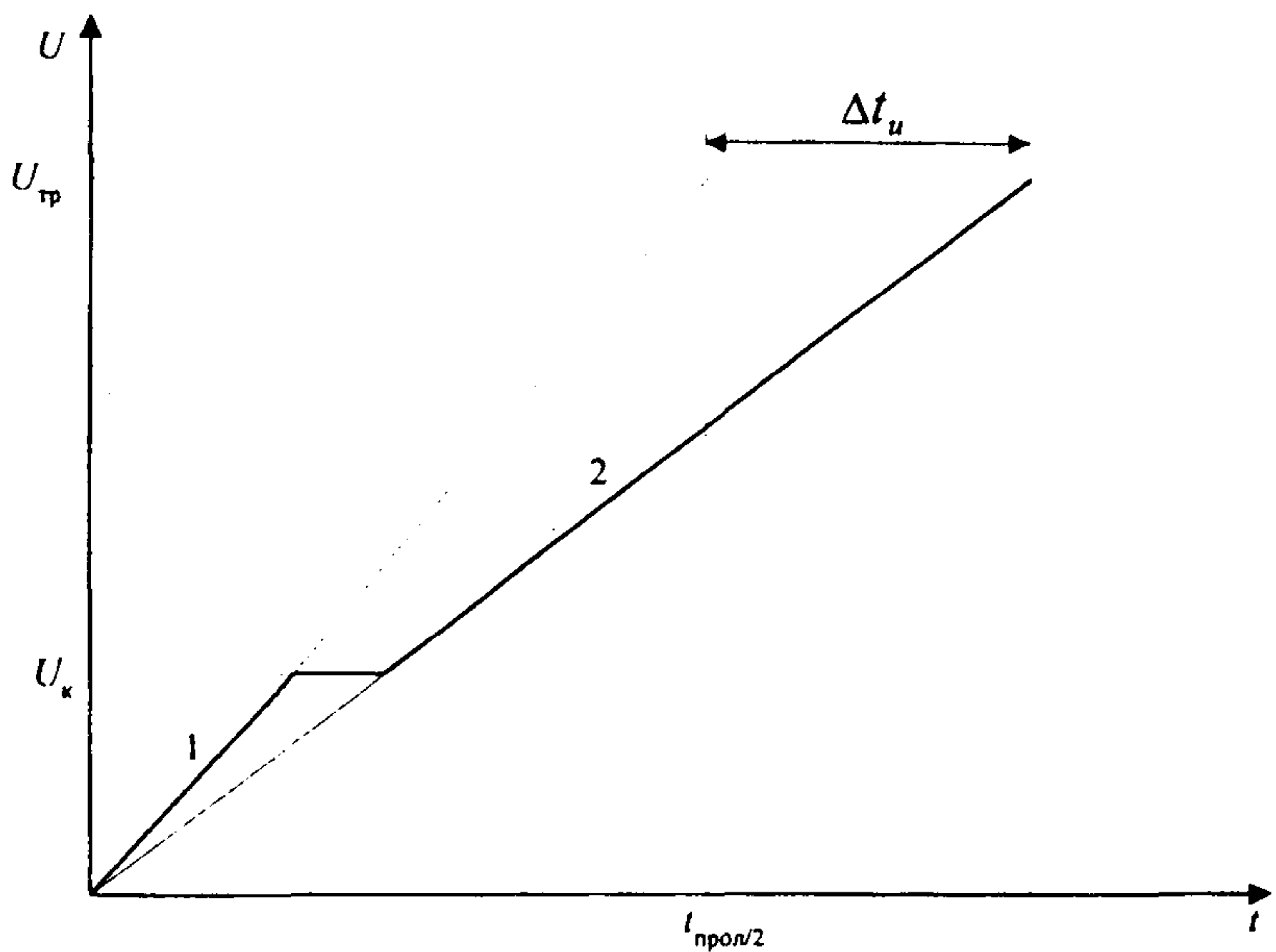
Рис. П17.4. Деформация фронта волны при пробеге по коронирующему тросу: 1 – фронт волны в середине пролета; 2 – деформированный фронт, определяющий крутизну импульсного тока через опору после пробеге волны
