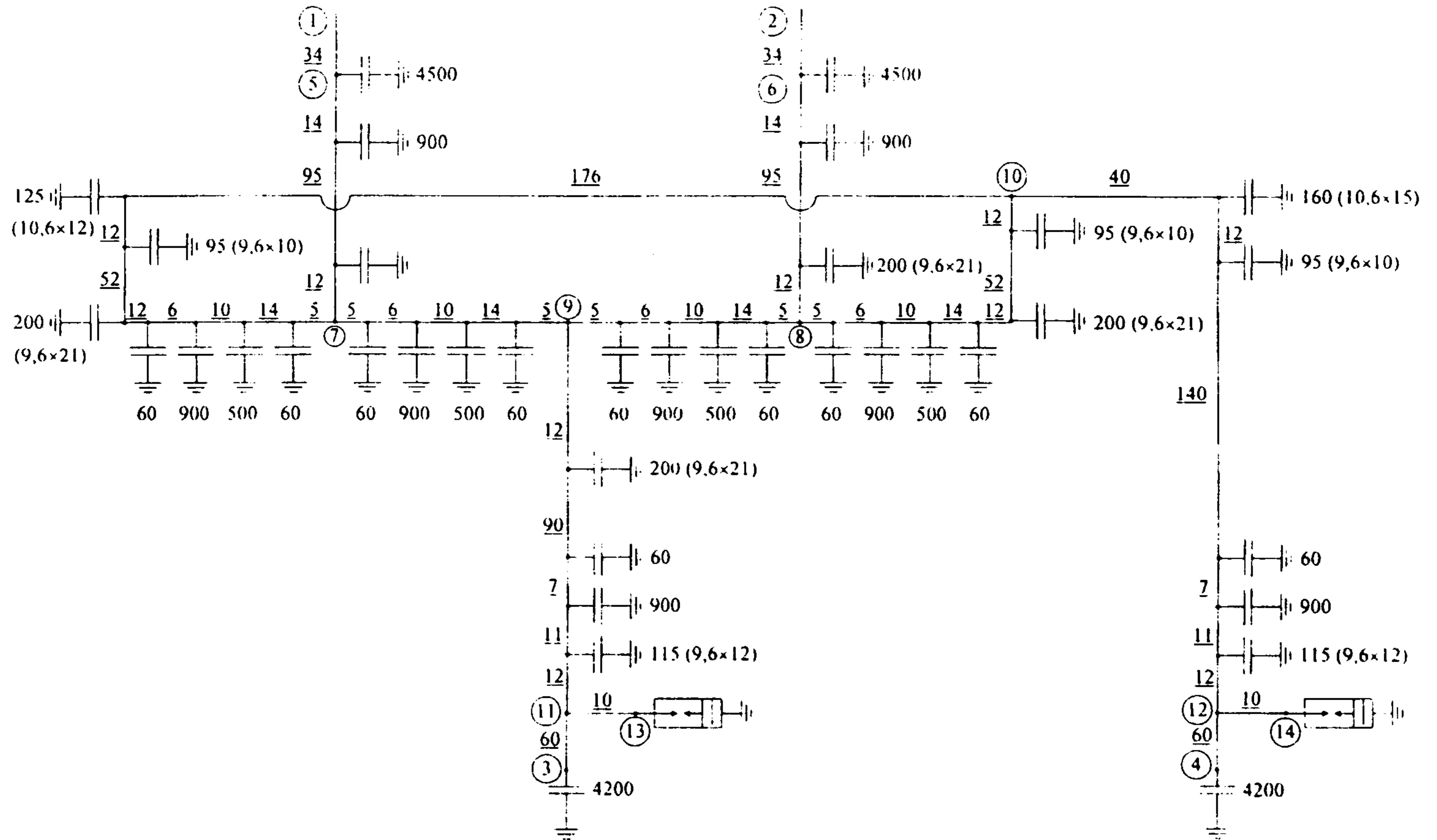
Рис 1130.8. Полная схема замещения ПС
