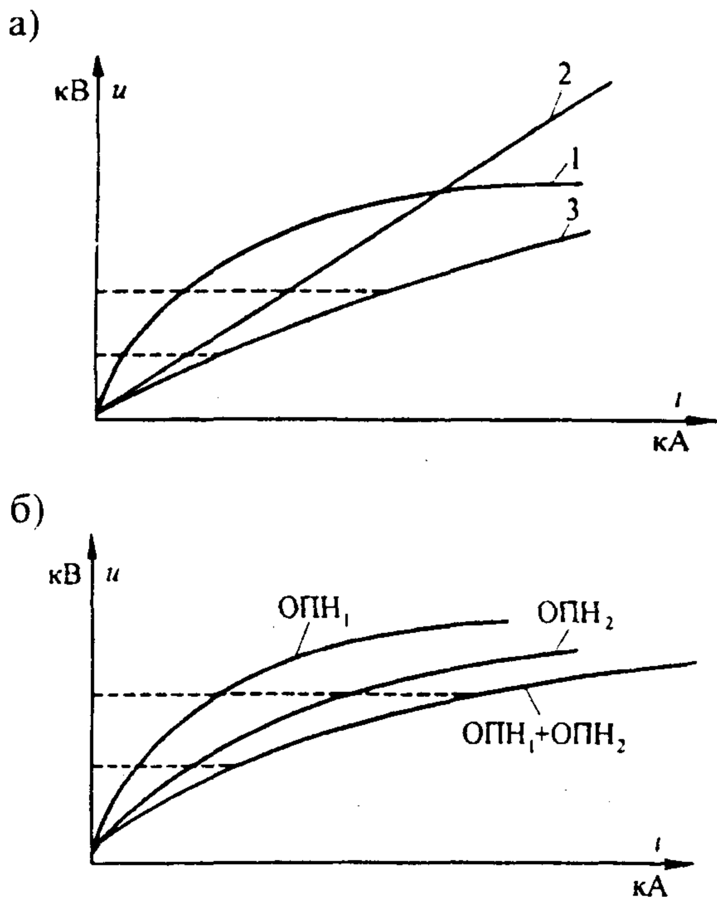
Рис. 9.3. Построение обобщающей вольт-амперной характеристики:
