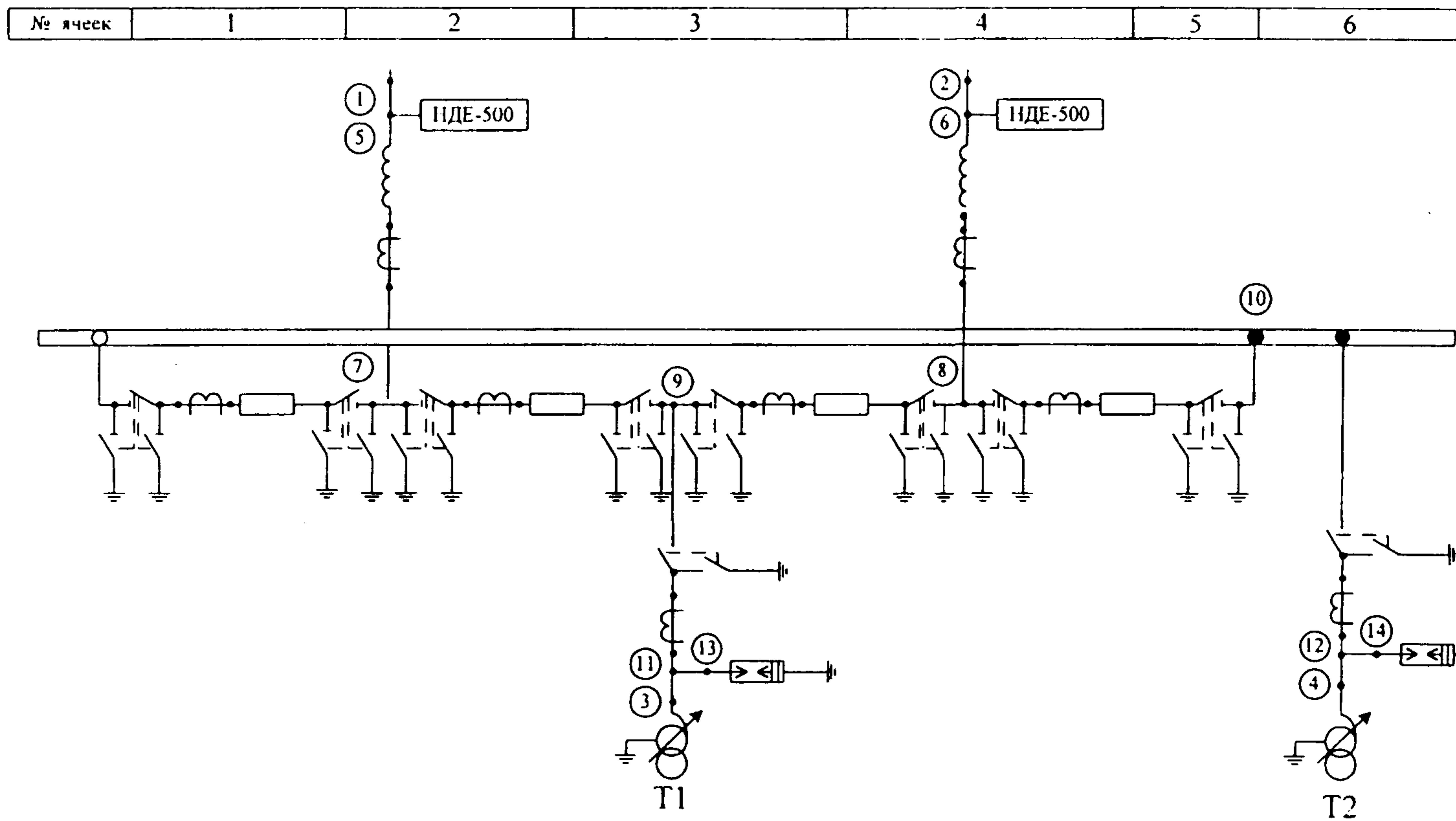
Рис. П30.1. Принципиальная схема ПС
