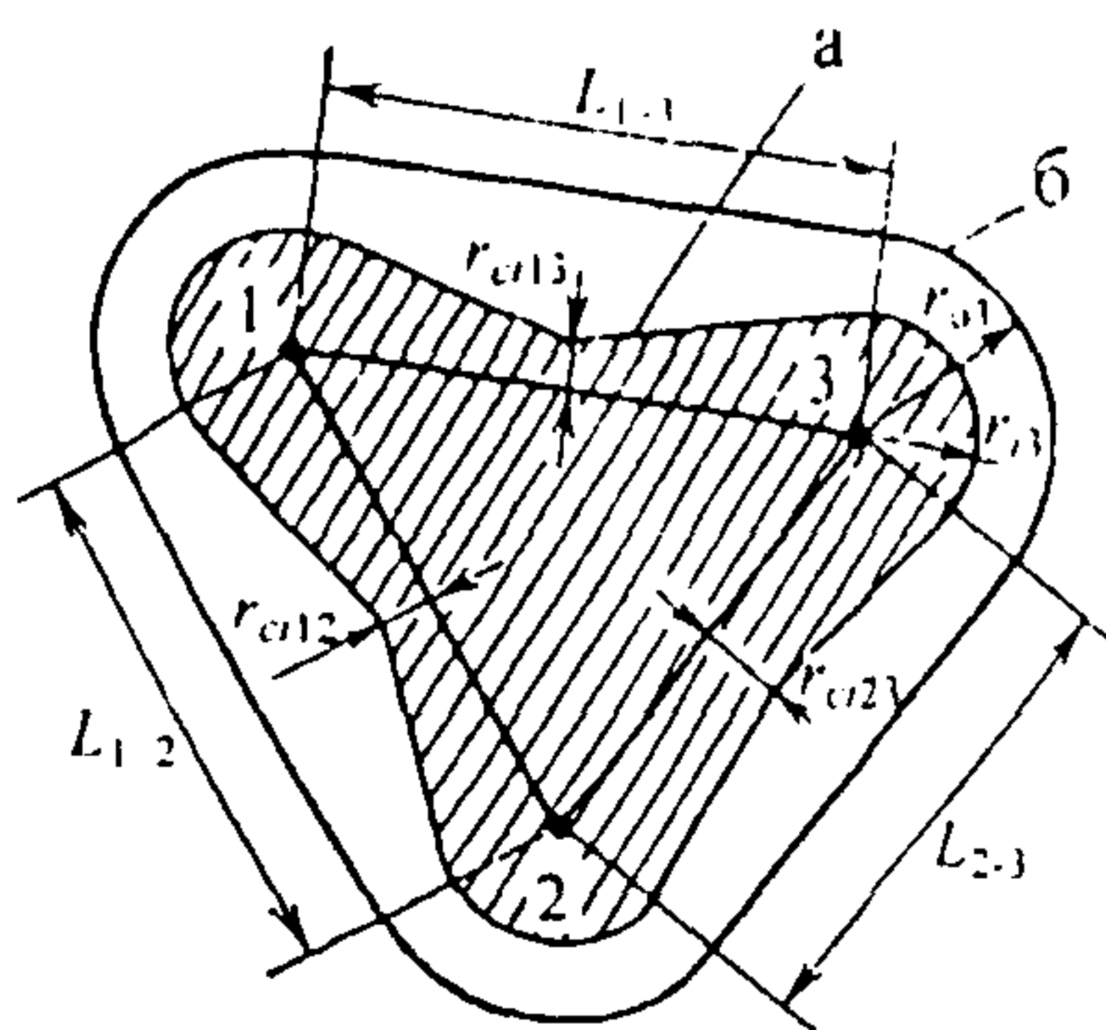
Рис. П29.4. Зоны защиты системы трех стержневых молниеотводов в плане: а - граница зоны защиты на уровне h_i ; б - то же, на уровне земли (при L_{м-м} \leq 2h )
