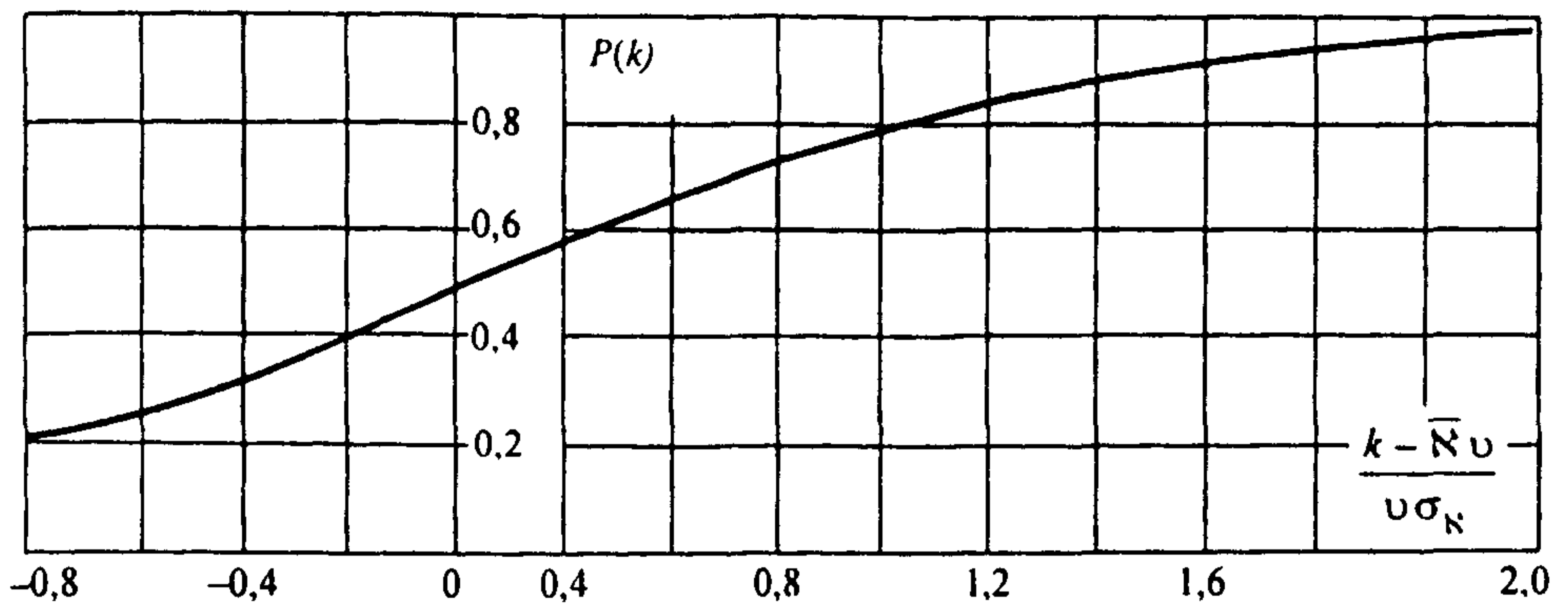
Рис. П6.5. Функция распределения амплитуд неограниченных перенапряжений ( U ; U_{н} ; U_{огтв} определяются по формуле (П6.7а) и по формулам Приложения 2)
