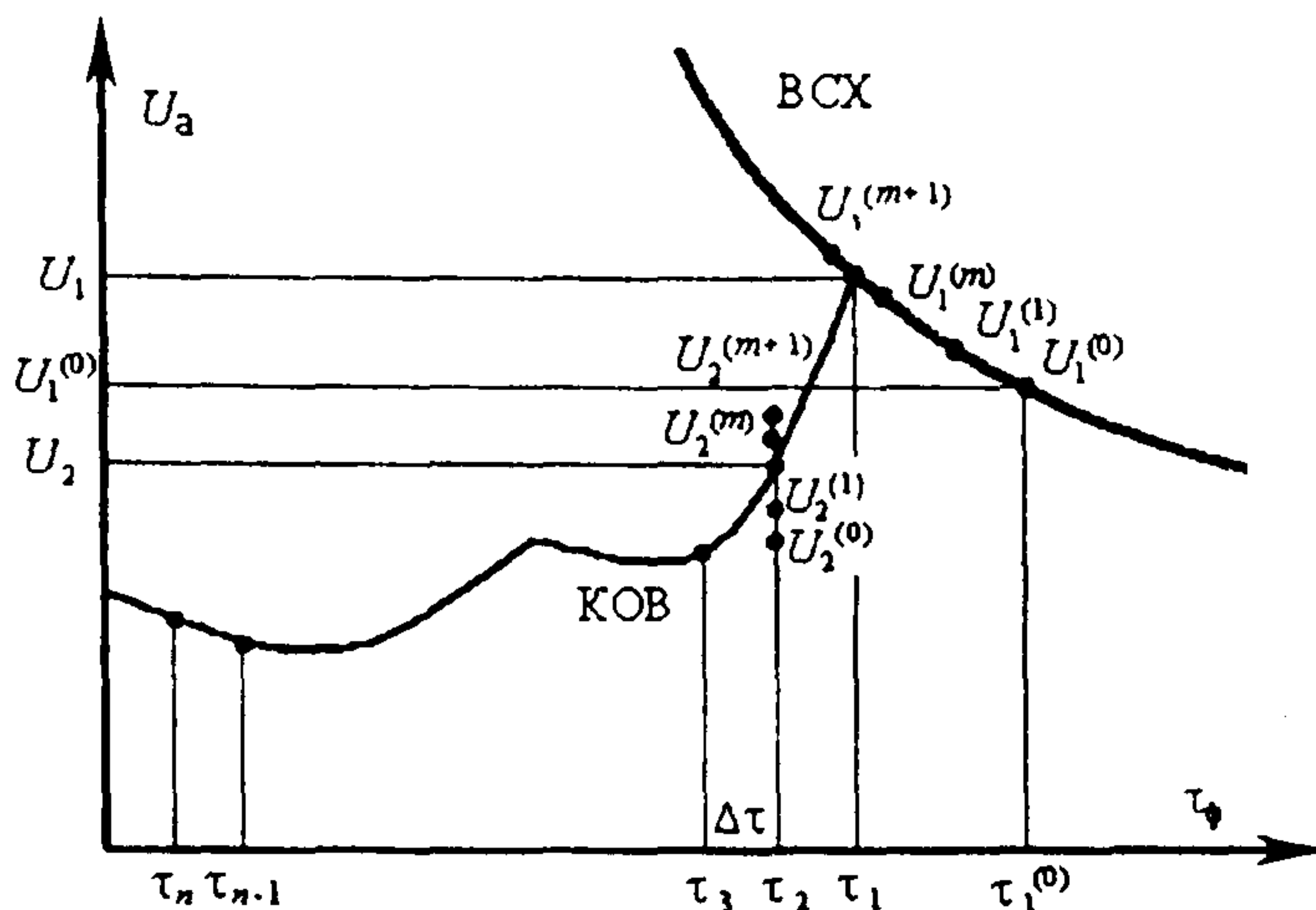
Рис. П33.4. Последовательность определения точек КОВ
