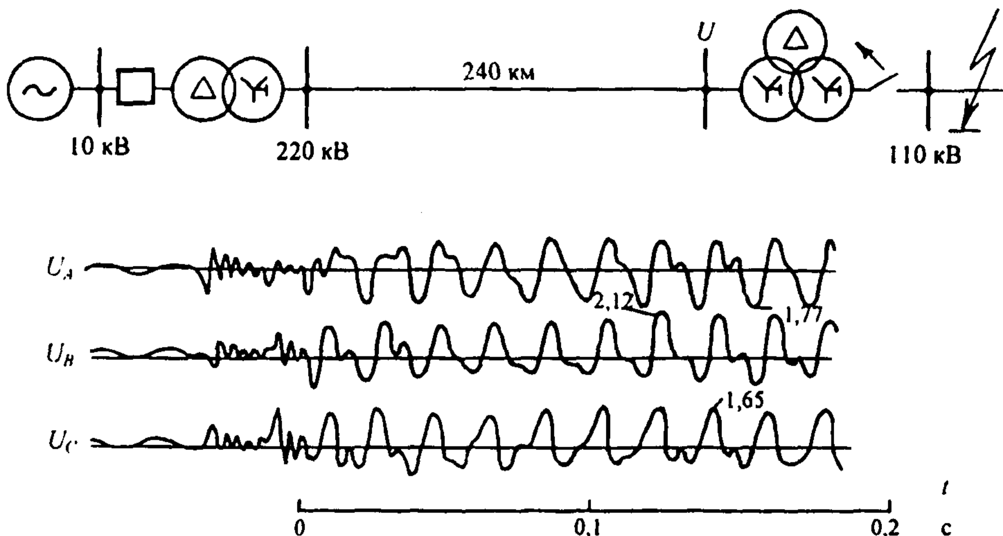
Рис. 2.3,б. Перенапряжения на частоте 100 Гц при переходном феррорезонансе на разомкнутом конце электропередачи 220 кВ Свирская ГЭС-Ленинград при отключении внешнего короткого замыкания
